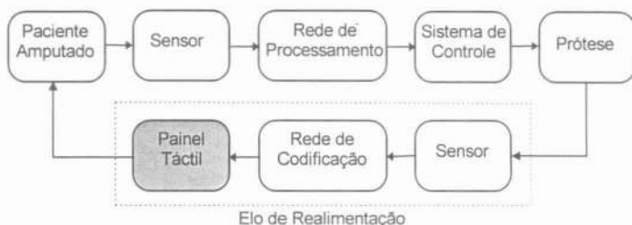
Figura 6. Diagrama de blocos de uma prótese realimentada sensorialmente.
