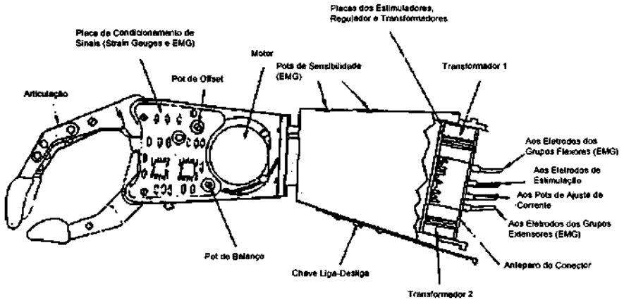
Figura 7. Exemplo de prótese de membro superior com realimentação sensorial de força de prensão, empregando eletrodos de superfície (de Prior et al. , 1976).
