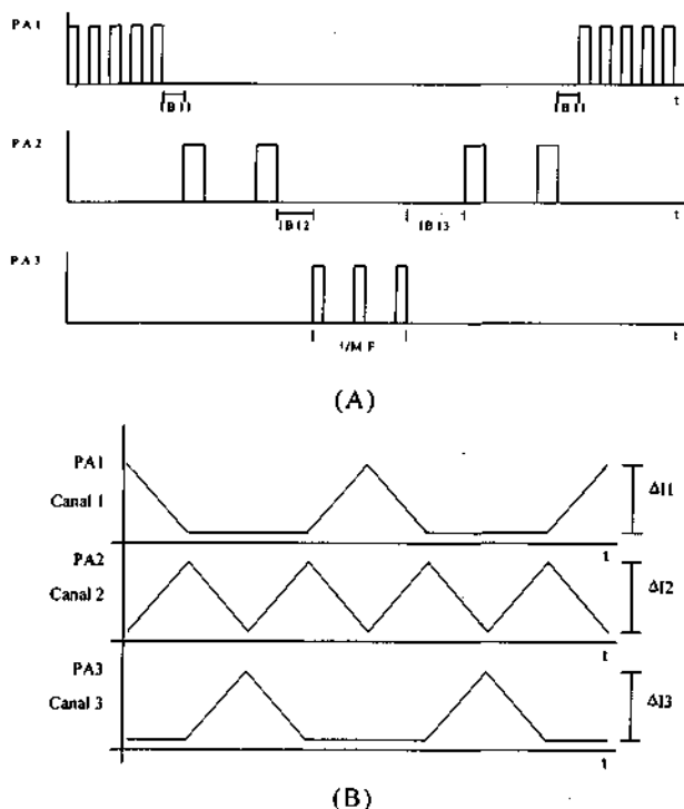
Figura 5. Relação de fase entre as correntes estimulatórias necessárias para evocação do fenômeno Phi táctil através das técnicas de: sequência de estímulos (A); e variação de amplitude com envoltória triangular (B); ambos para três canais. PA representa a amplitude máxima dos pulsos de corrente; \Delta I representa a variação da corrente estimulatória; IBI corresponde ao intervalo interbursts e 1/MF , o período do sinal modulante.
